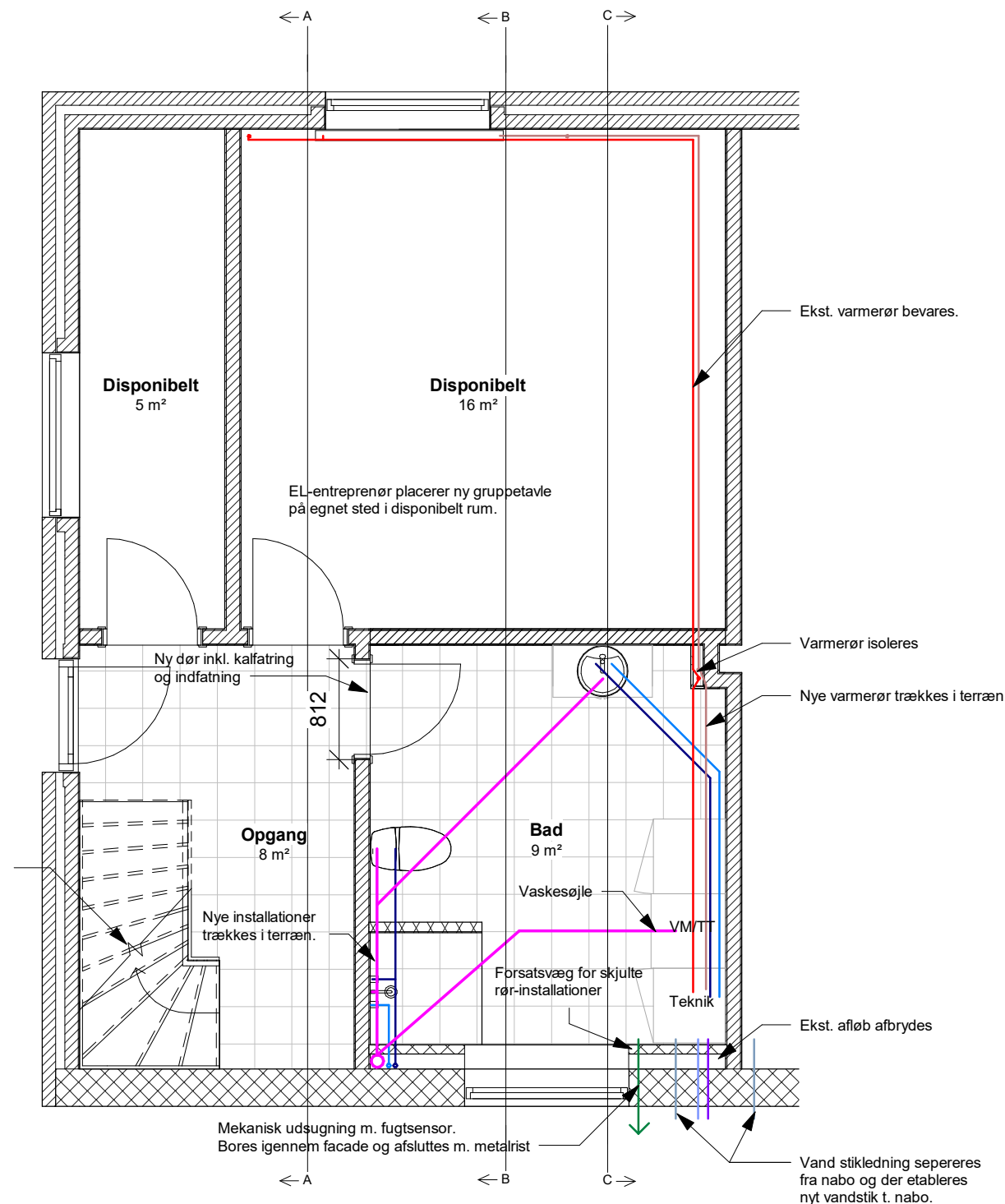
-01 - Kælderplan | 1 : 50
